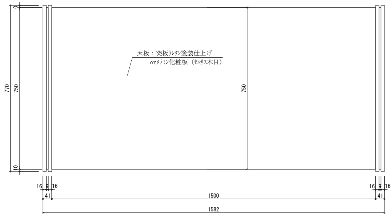
平面図
